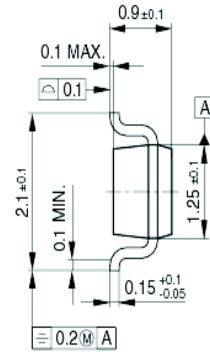
SOT343-PO V08
