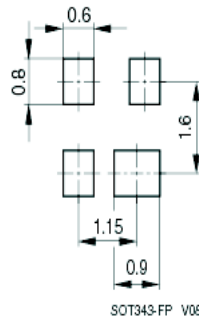
SOT343-FP V08
