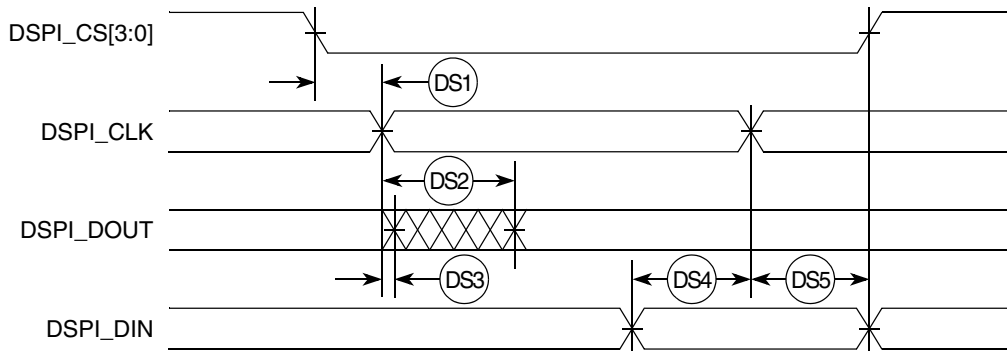
Figure 30. DSPI Timing
