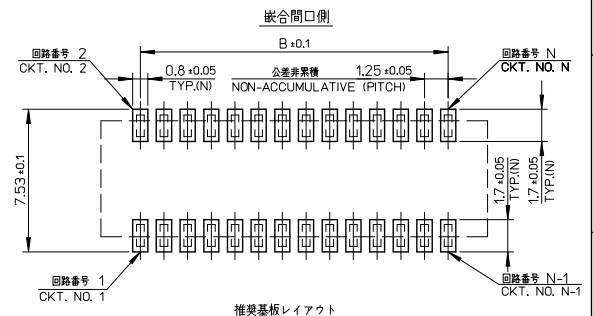
推奨基板レイアウト
