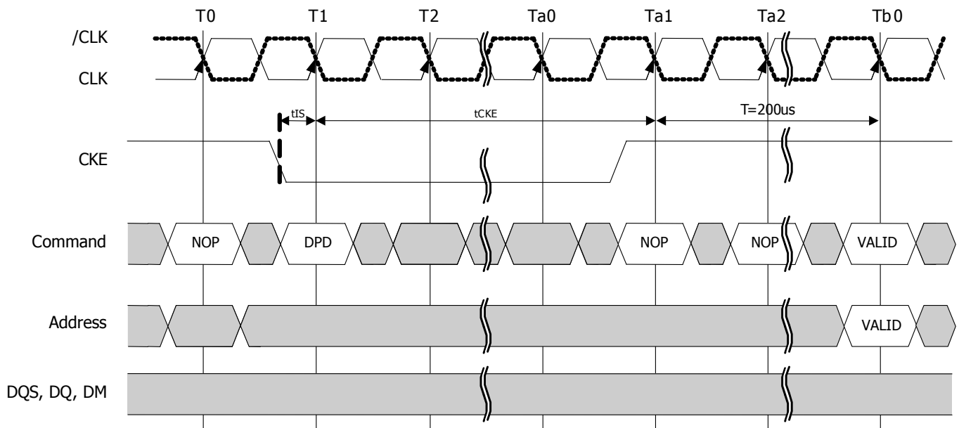
Figure36 : Deep Power down
