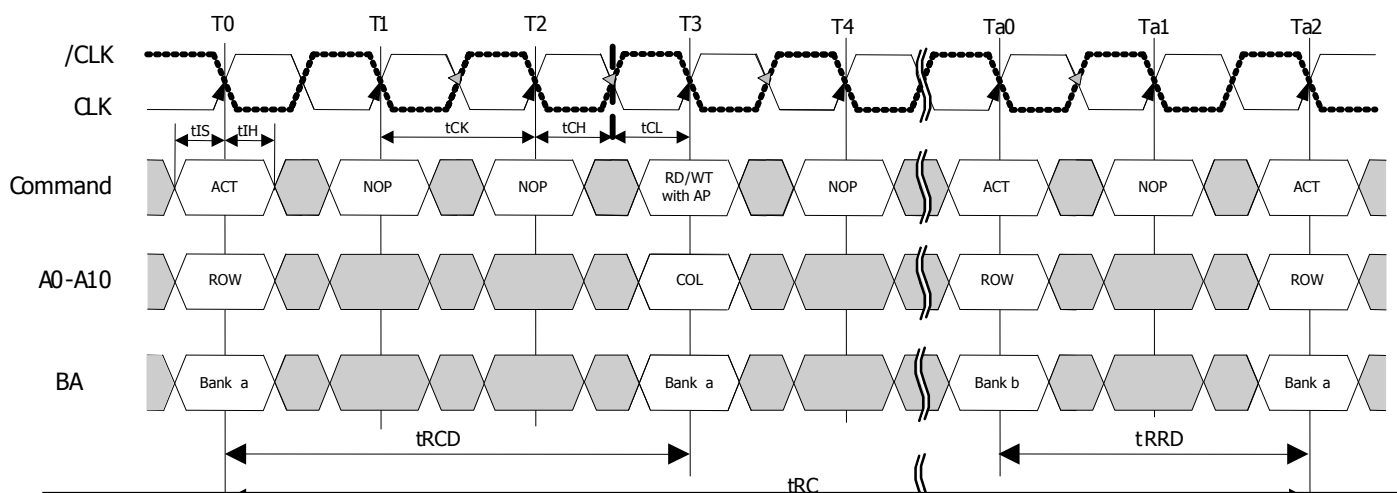
Figure11 : tRCD, tRRD, tRC
