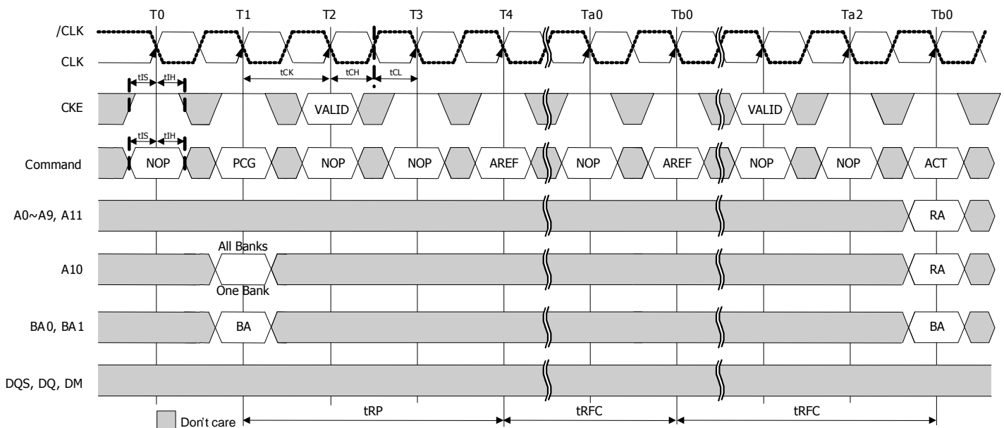
Figure33 : Auto refresh
