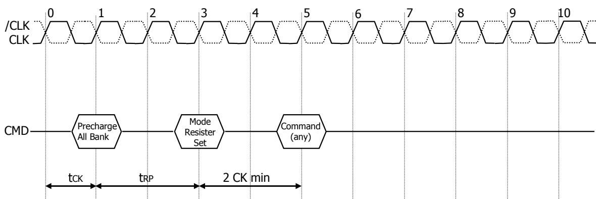
Figure32 : Mode Resister Set
