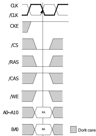
Figure10 : Active command
