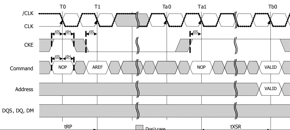
Figure34 : Self refresh
