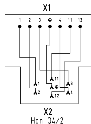
Schaltplan/wiring plan
