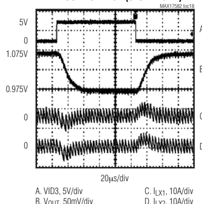
VID CODE CHANGE (SLOW = GND)
